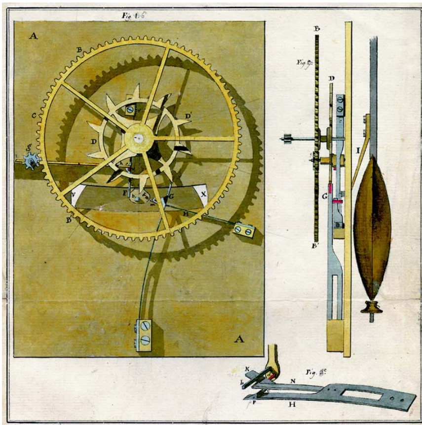
Patente del invento de Abraham-Louis Bregue, registrado el 9 de marzo de 1798 Mecanismo de relojería llamado escape de fuerza constante Papel. 0,365 x 0,555 x 0,01 cm. Paris, Instituto Nacional de la Propiedad Industrial, inv. 1BA146 © Instituto Nacional de la Propiedad Industrial
